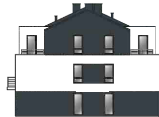
Elewacja południowa
