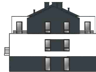
Elewacja południowa
